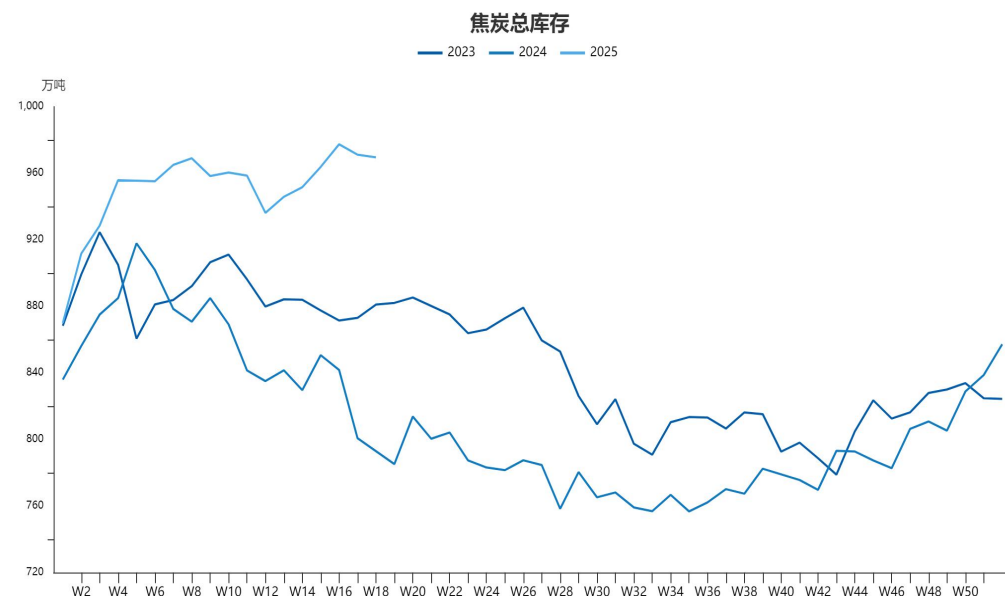
图12、焦炭总库存
