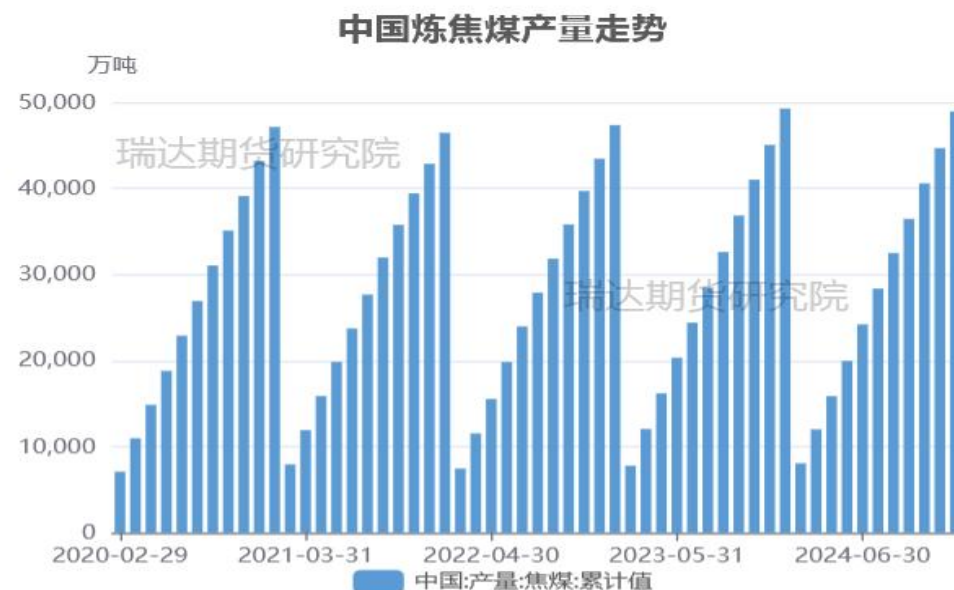
图8、炼焦煤产量
